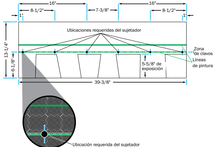
PATRÓN DE SUJECIÓN EN TECHO ABUHARDILLADO O PENDIENTE PRONUNCIADA
